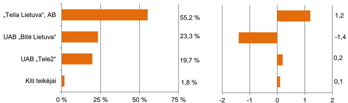
65 pav. SIM kortelių, naudojamų M2M paslaugoms teikti, skaičiaus dalis pagal paslaugų teikėjus, proc., ir rinkos dalių metiniai pokyčiai, proc. punktais, 2020 m.
