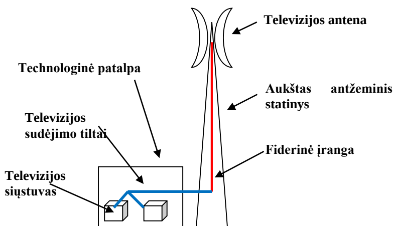
10 pav. DVB-T transliacijų perdavimo priemonės kartu su siūstuvais schema Šaltinis: RRT
