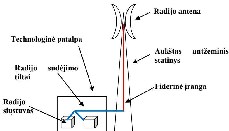
15 pav. Radijo priemonės, kartu su radijo siųstuvais, schema Šaltinis: RRT
