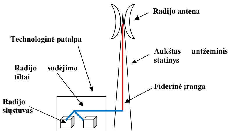
15 pav. Radijo priemonės, kartu su radijo siūstuvais, schema Šaltinis: RRT
